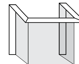
Rama montażowa 5-stronna szerokość 70 mm grubość 4 mm
